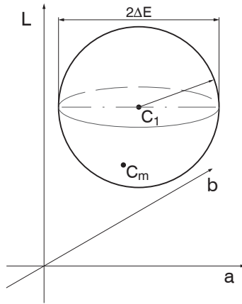
Abb. 2 Toleranzraum Kugel
