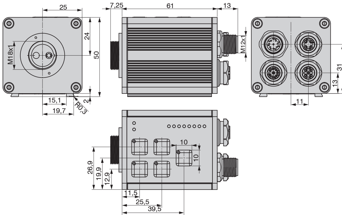
Abb. 6 Maßzeichnung colorSENSOR CFO100/CFO200/CFO250, Abmessungen in mm
