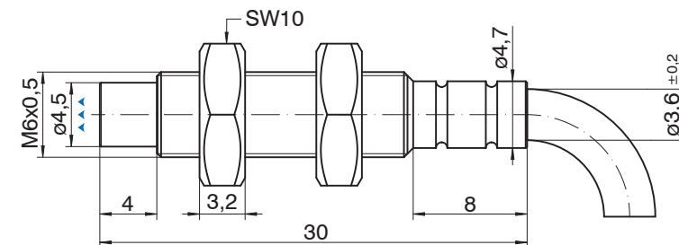
Abb. 5 ES-U1-C-CAx, Abmessungen in mm (nicht maßstabsgetreu)
