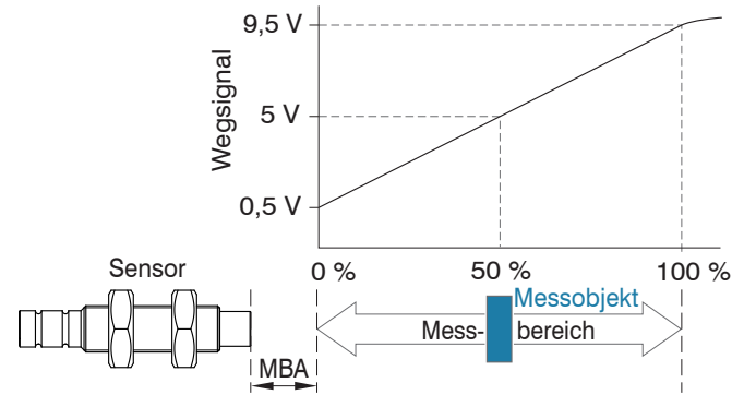
Abb. 1 Messbereichsanfang (MBA), der kleinste Abstand zwischen Sensorstirnfläche und Messobjekt
