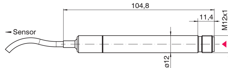
Abb. 6 DT3005-x, Abmessungen in mm (nicht maßstabsgetreu)
