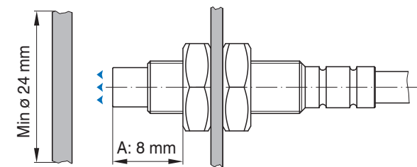
Abb. 2 Montage, Abmessungen in mm (nicht maßstabsgetreu)
