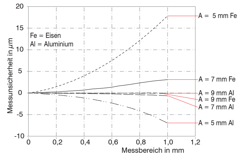
Abb. 3 Messunsicherheit in Abhängigkeit von Abstand A und Messobjektmaterial
