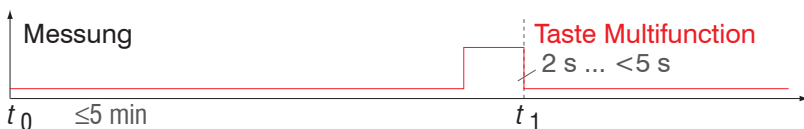
Abb. 65 Ablaufdiagramm für die Rücknahme Nullsetzen, Mastern
