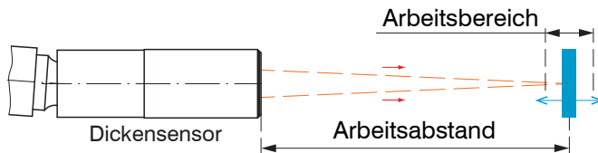
Abb. 3 Dickensensor IMP-THxx mit Arbeitsabstand und Arbeitsbereich
