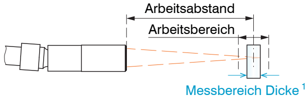
Abb. 34 Grundlagen Dickenmessung
