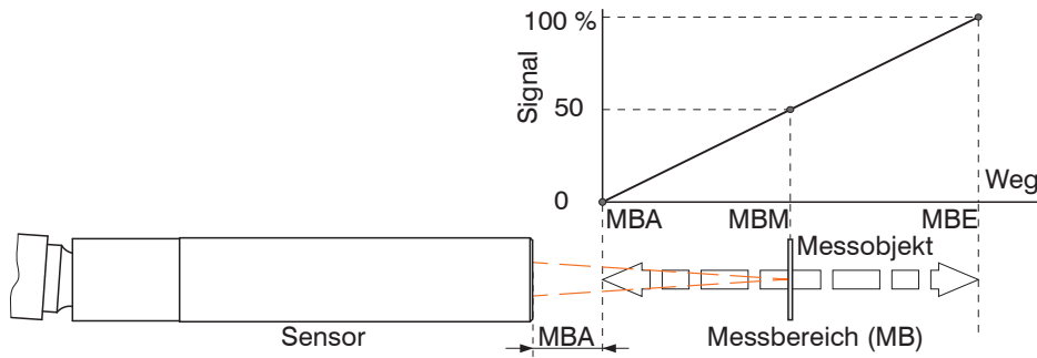
Abb. 2 Abstandssensor IMP-DS, Messbereich und Ausgangssignal am Controller
