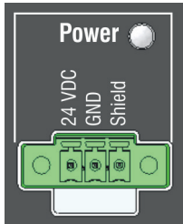
Abb. 11 Versorgungs-Anschlüsse und LED am Controller IMC5x00
