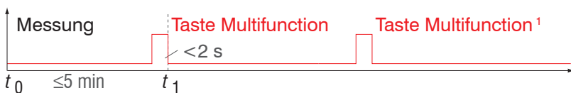
Abb. 64 Ablaufdiagramm für Nullsetzen, Mastern (Taste Multifunction)
