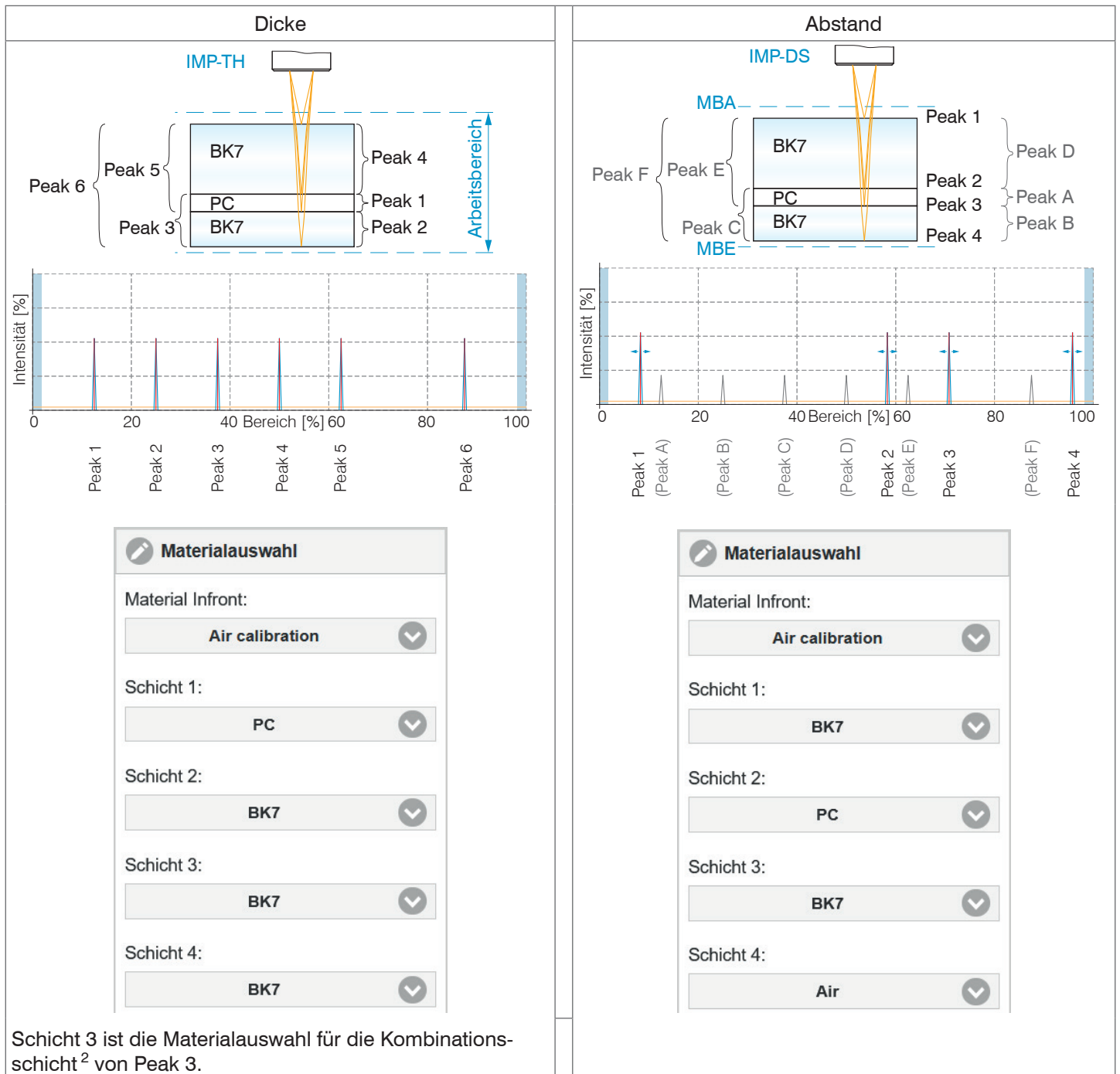
Abb. 48 Messanordnung aus drei Schichten mit zugehöriger Materialauswahl
