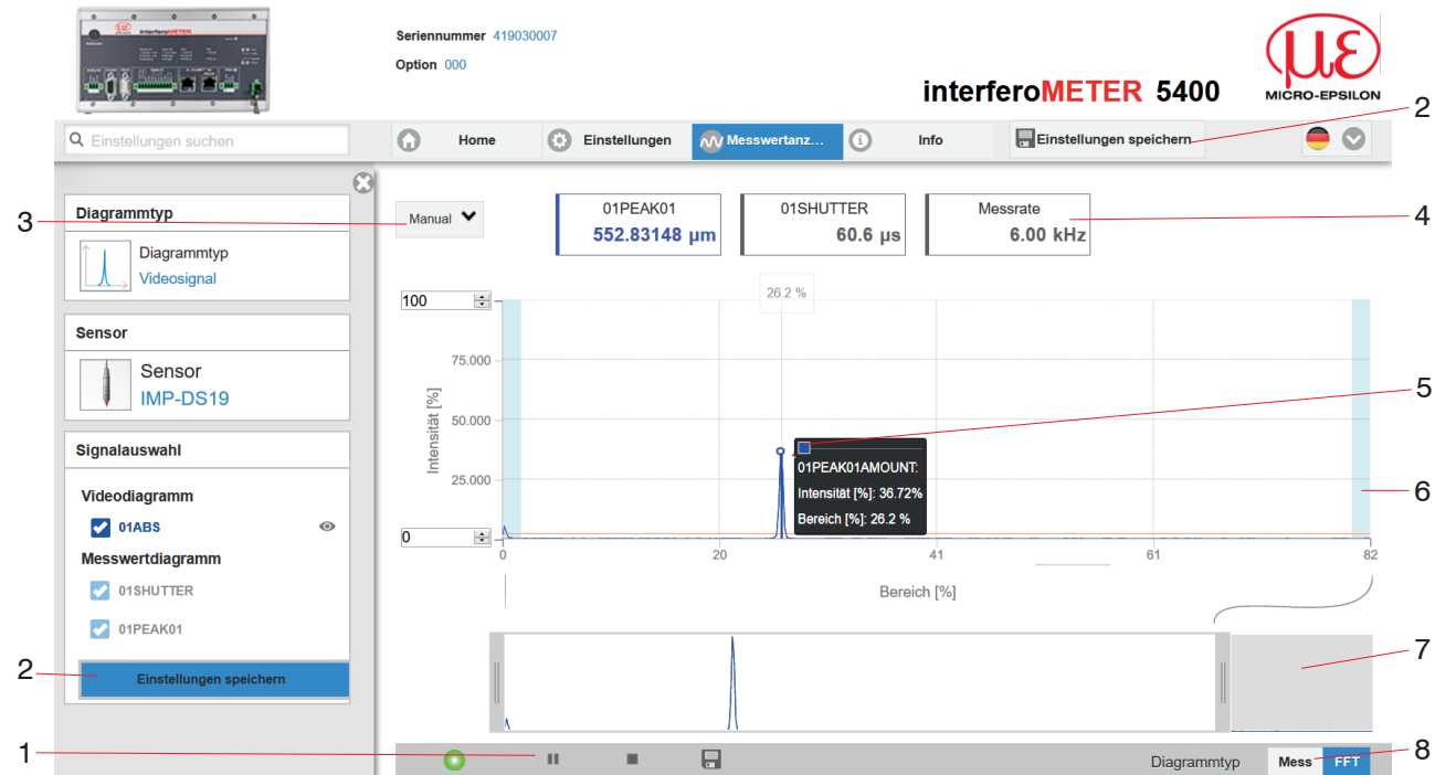
Abb. 35 Webseite FFT-Signal
