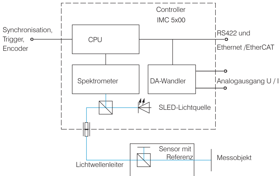
Abb. 1 Blockschaltbild IMS5x00-DSxx
