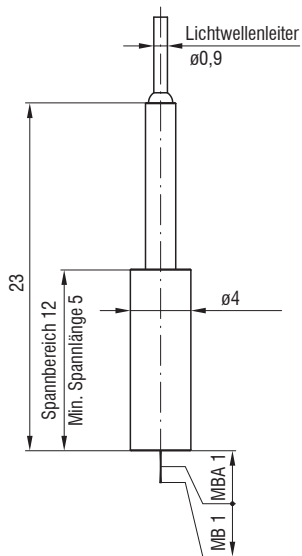
Abb. 22 Abstandssensor IMP-DS1/VAC
