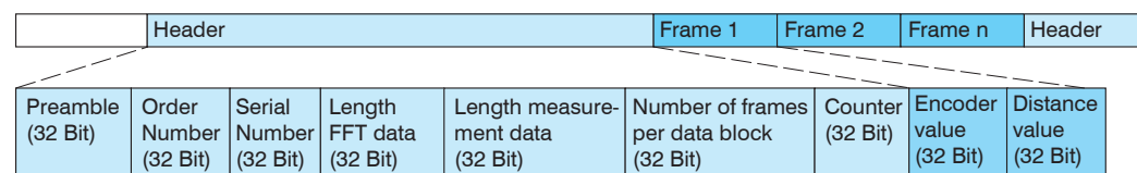
Abb. 78 Beispiel für eine Datenübertragung mit Ethernet
