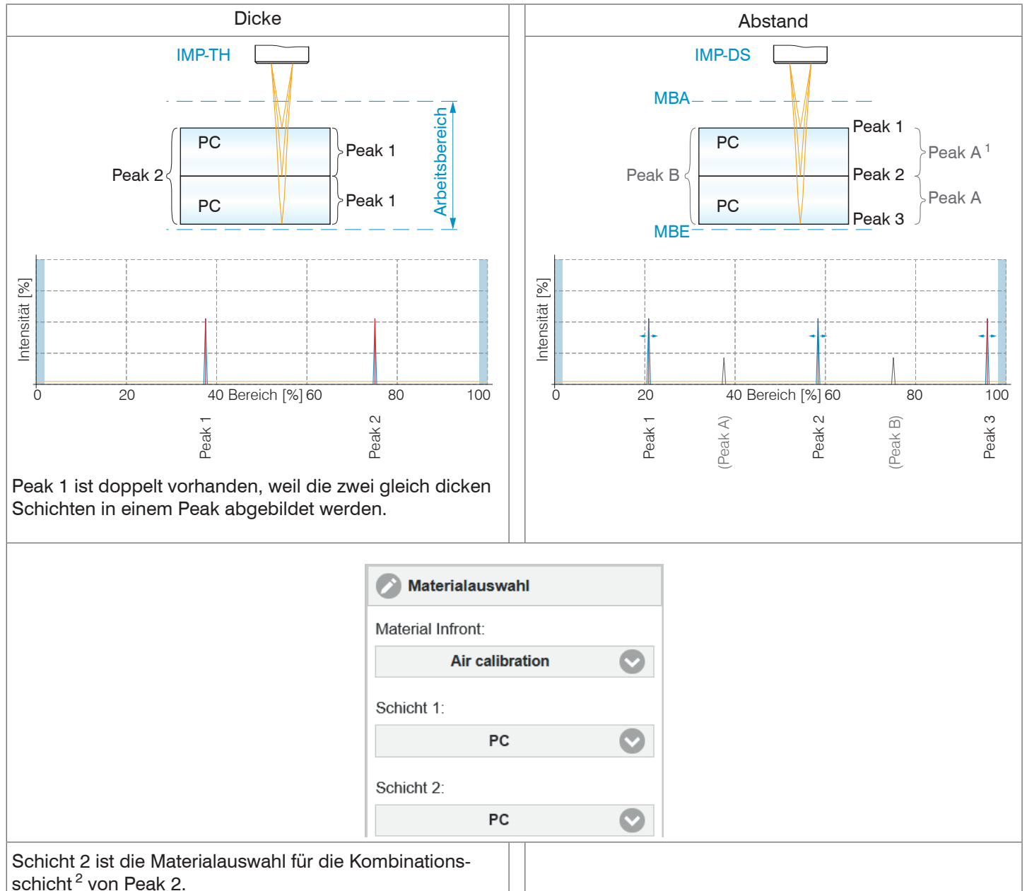
Abb. 49 Messanordnung aus zwei Schichten mit gleicher Dicke und zugehöriger Materialauswahl
