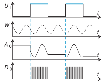
Abb. 51 Triggerung mit aktivem High-Pegel ( U_1 ), zugehöriges Analogsignal ( A_0 ) und Digitalsignal ( D_0 )
