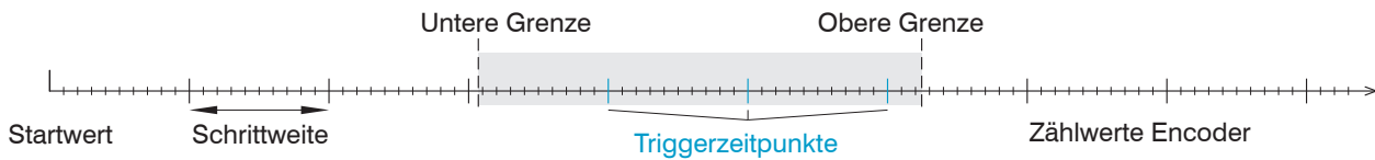
Abb. 53 Begriffsdefinition für die Encoder-Triggerung
