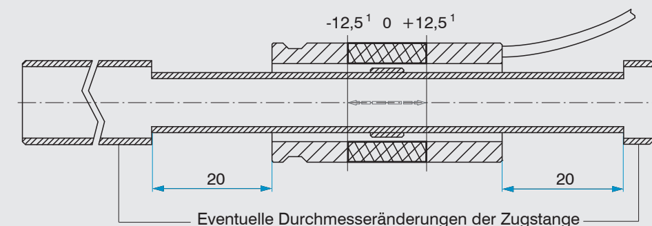
Abb. 8 Abmessungen Zugstangenanschluss, am Beispiel LVP-25-Z20
