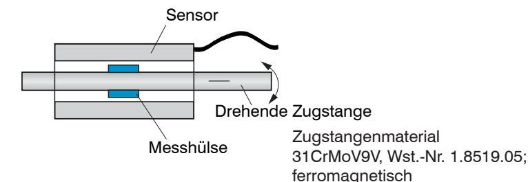
Abb. 5 Zugstange mit Sensor
