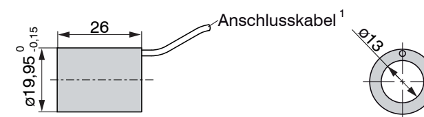
Abb. 3 Abmessungen des LDR-14-Z20, Abmessungen in mm, nicht maßstabsgetreu
