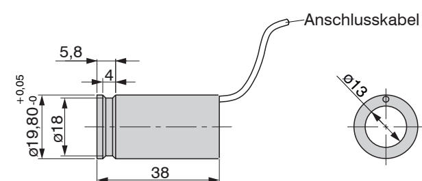
Abb. 2 Abmessungen des LVP-25-Z20, Abmessungen in mm, nicht maßstabsgetreu
