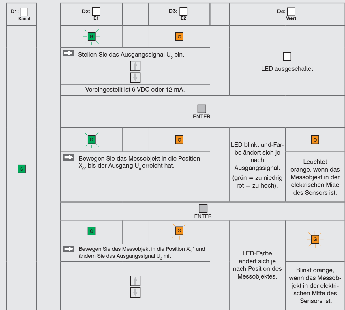
Abb. 9 Menüstruktur Controller MSC7401, Justagemodus: Null-Punkt-Suche
