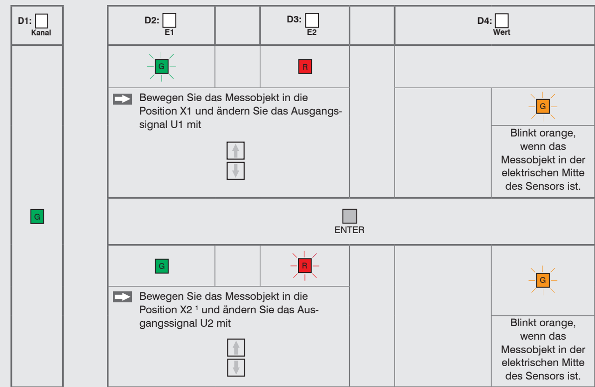
Abb. 8 Menüstruktur Controller MSC7401, Justagemodus: 2-Punkt-Abgleich
