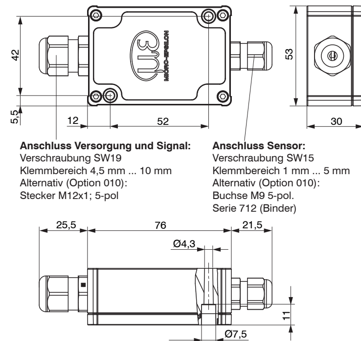
Abb. 1 Abmessungen des Controllers MSC7401 1 , Abmessungen in mm, nicht maßstabsgetreu 1) Option induSENSOR MSC7401 (010) hat unterschiedliche Abmessungen.
