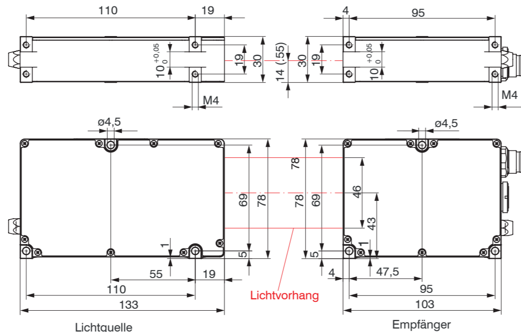
Abb. 1 Maßzeichnung Lichtquelle und Empfänger, Abmessungen in mm, nicht maßstabsgetreu
