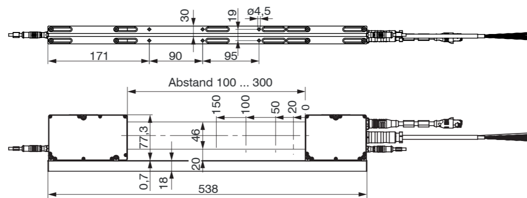
Abb. 2 Maßzeichnung Lichtquelle und Empfänger mit Montagesschiene, Abmessungen in mm, nicht maßstabsgetreu
