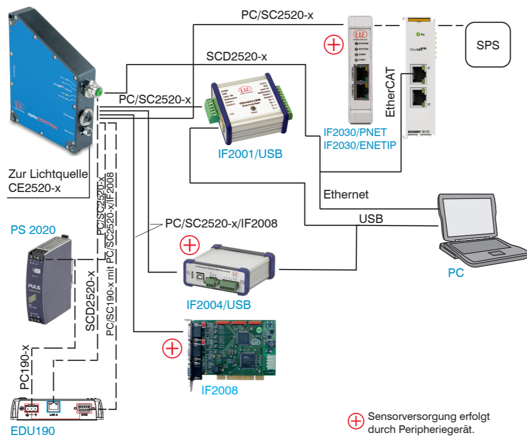
Abb. 6 Anschlussbeispiele am optoCONTROL 2520-95
