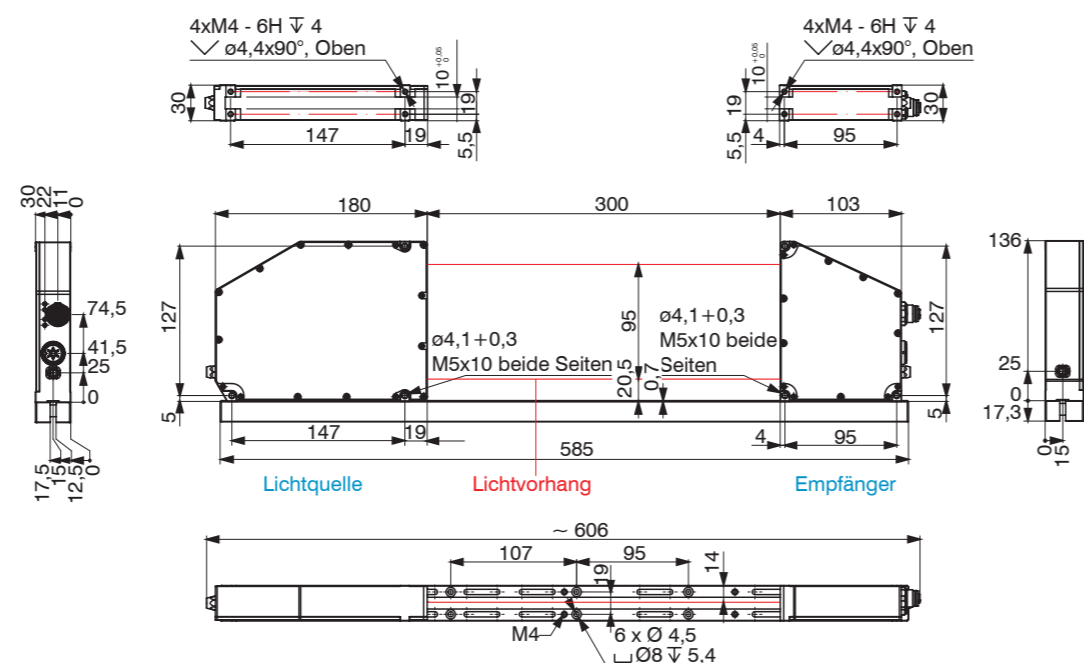
Abb. 1 Maßzeichnung Lichtquelle und Empfänger mit Montageschiene 1 , Abmessungen in mm, nicht maßstabsgetreu
