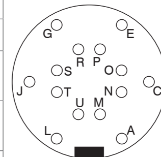
14-pol. Kabelstecker Ansicht Lötseite
